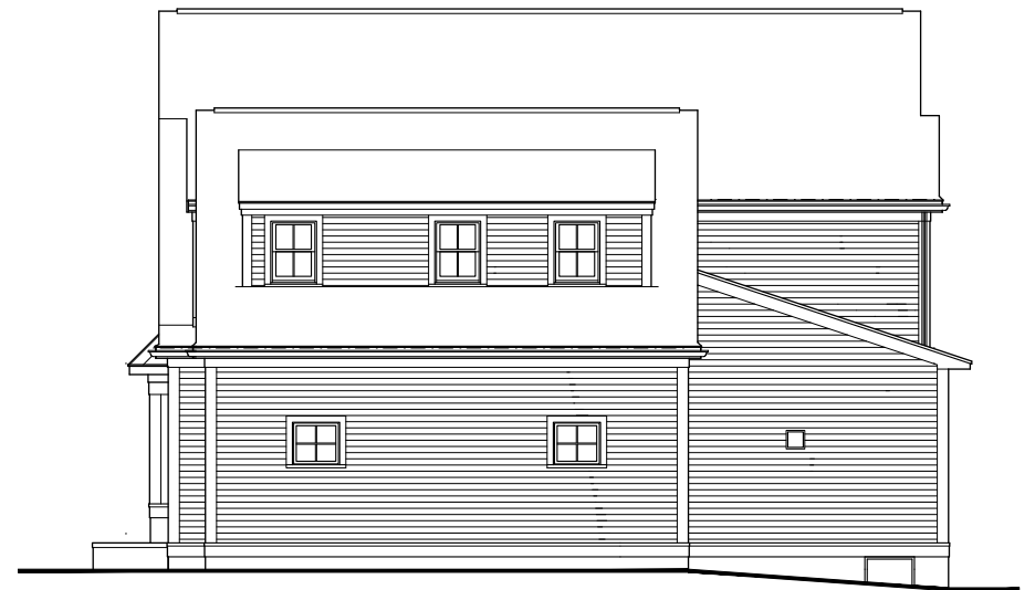
Right Elevation
